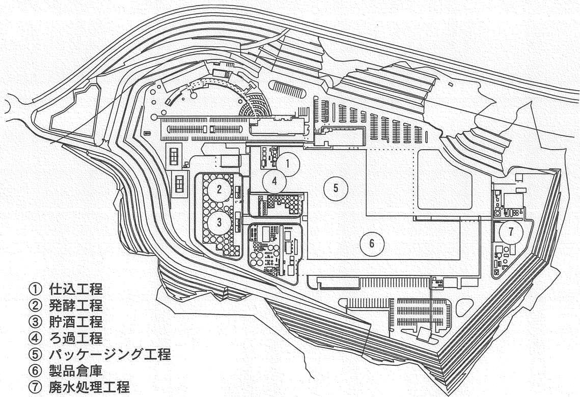
図3 工場配置図
