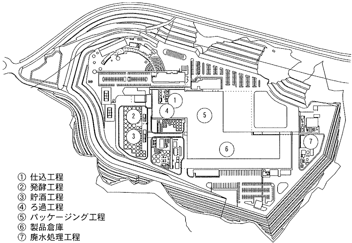
図3 工場配置図
