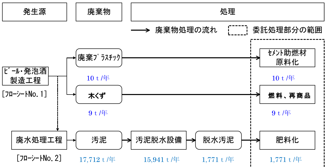
図4 廃棄物処理フローシート ※発生量は、平成29年度実績
