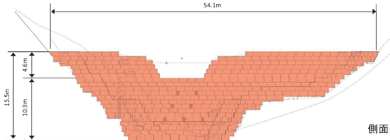
正面図
