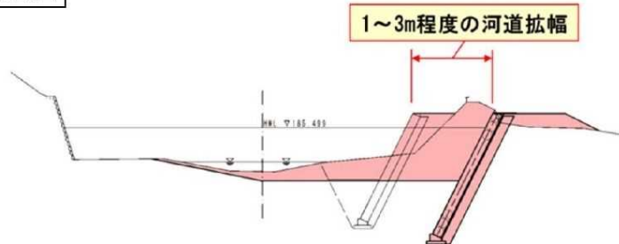
横断面図
