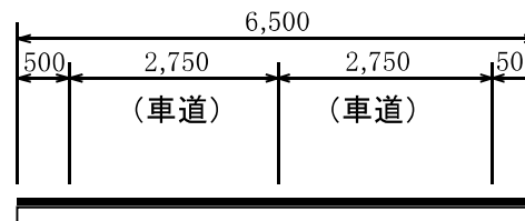
【単位:mm】
